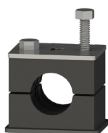
1 collier, 1 plaque à souder, 1 plaque supérieure, 2 vis CHC
