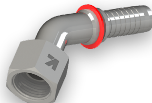
Type B : Écrou rapporté
