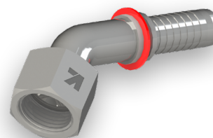
Type B : Écrou rapporté
